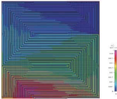
氫氣流道濃度分佈
