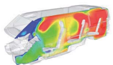
車內溫度控制
