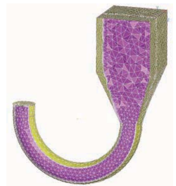
非結構網格應用於管內流
